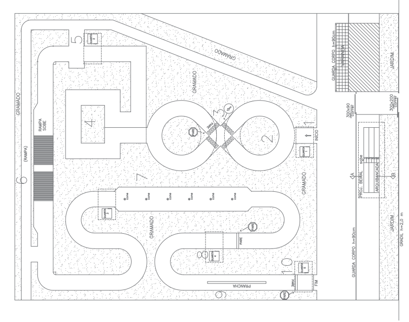
LAYOUT – PISTA DE MOTO ESCALA 1/200
